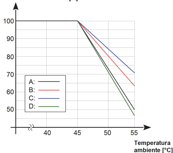
Derating coppia erogata rispetto al valore nominale [%]
